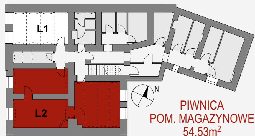
USYTUOWANIE POM. MAGAZYNOWEGO W BUDYNKU
