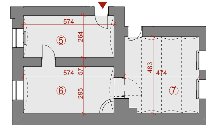
POGLĄDOWY RZUT POM. MAGAZYNOWYCH
